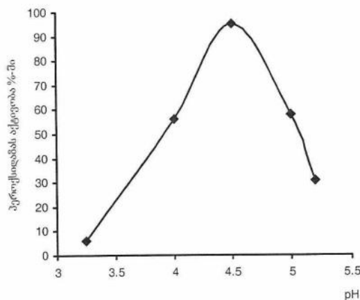
სურ.3 ქერის ალაოს პეროქსიდაზას აქტივობის დამოკიდებულება PH-ზე.
