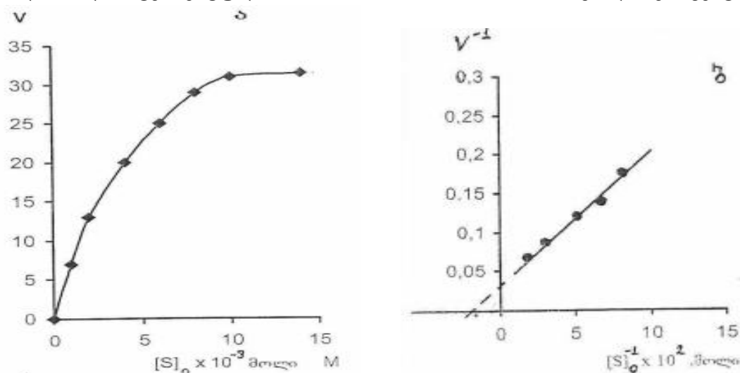
სურ.1 გვიაკოლის კონცენტრაციის გავლენა პეროქსიდაზას აქტივობაზე ა-კოორდინატებში V-[S]_0 , ბ- ლაინუვერ-ბერკის კოორდინატებში.
